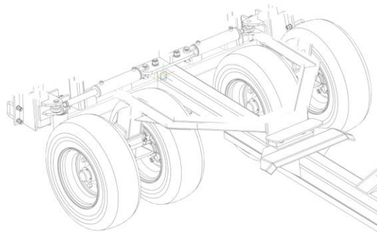
Рисунок 18. Расположение фитингов для выпуска воздуха в системе складывания
