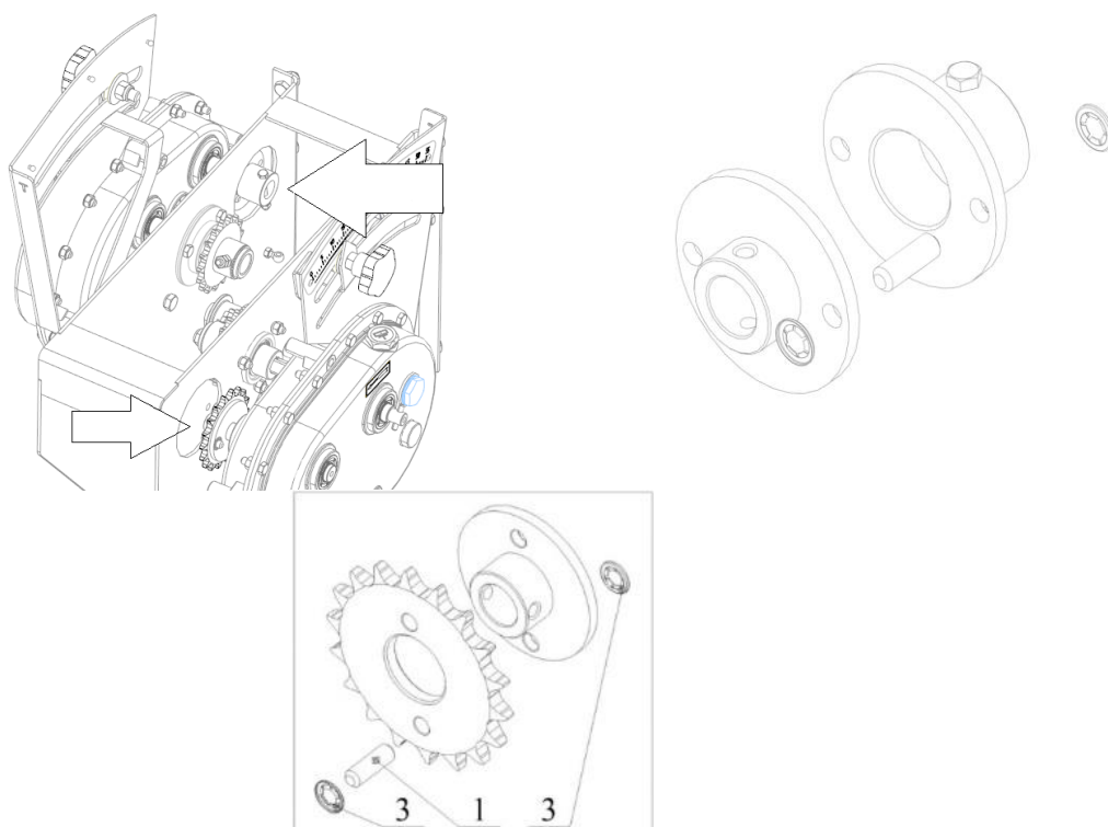
Рисунок 27. Размещение и устройство предохранительных муфт. 1- предохранительный полимерный штифт. 3 – шайба starlock
