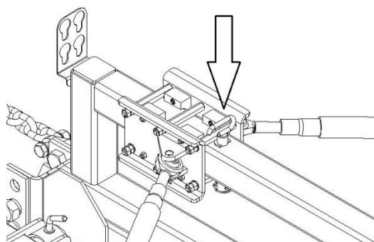
Рисунок 23. Палец тяговой штанги в трансп. положении
