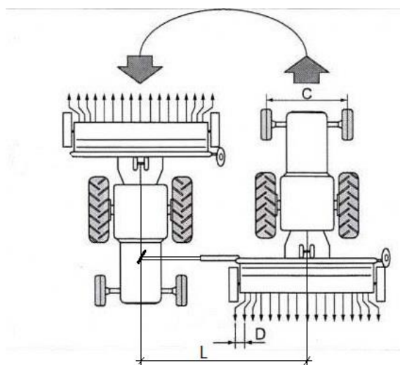
Рисунок 14. Расчётная схема настройки вылета маркеров
