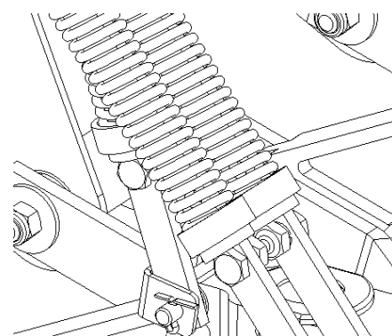
Рисунок 13. Болты нижних стаканов пружин
