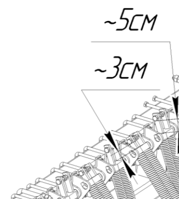
Рисунок 20. Вылеты концов штанг передних и задних секций
