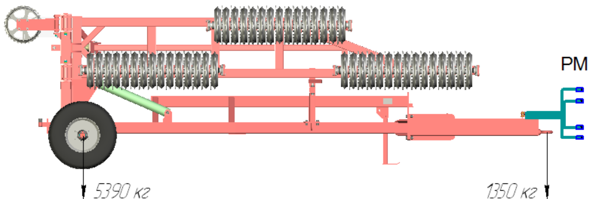
Рис. 8 Распределение веса катка
