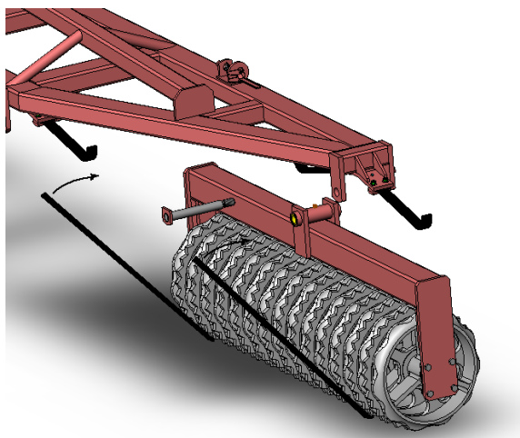
Рис.7 Установка секции катка с помощью ручных приспособлений
