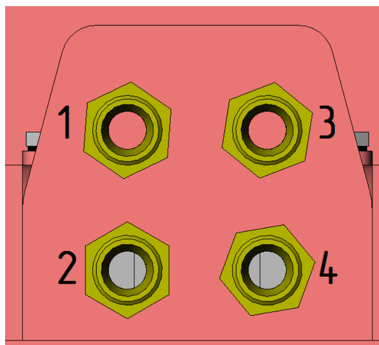
Рис. 9 Схема подключения гидравлических шлангов к катку
