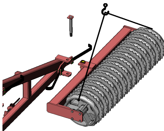
Рис.6 Установка секции катка с помощью подъемного механизма
