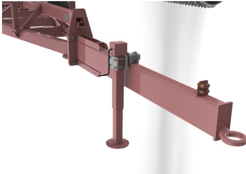
Рис. 13 Установка домкрата в рабочее положение
