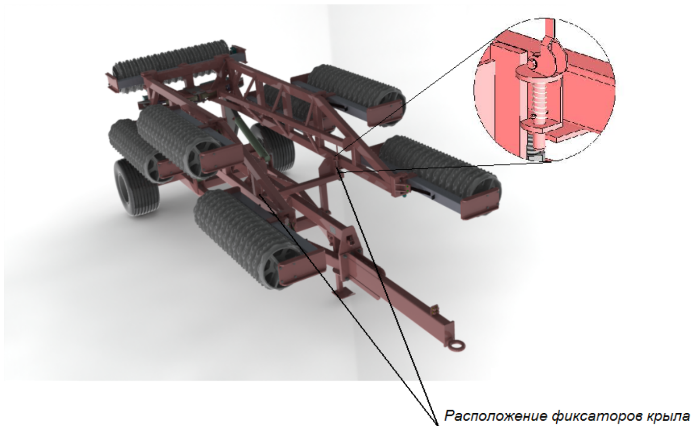
Рис. 10 Расположение фиксаторов на раме катка
