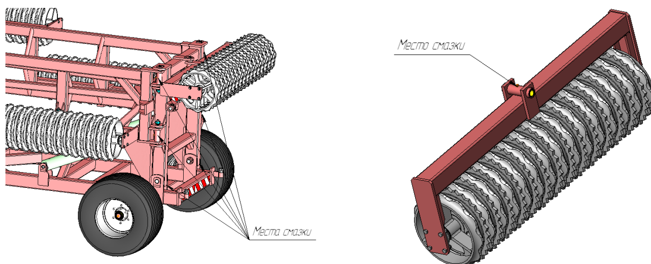
Рис.15 Места смазки
