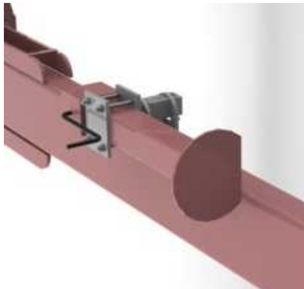
Рис. 14 Установка домкрата в транспортное положение
