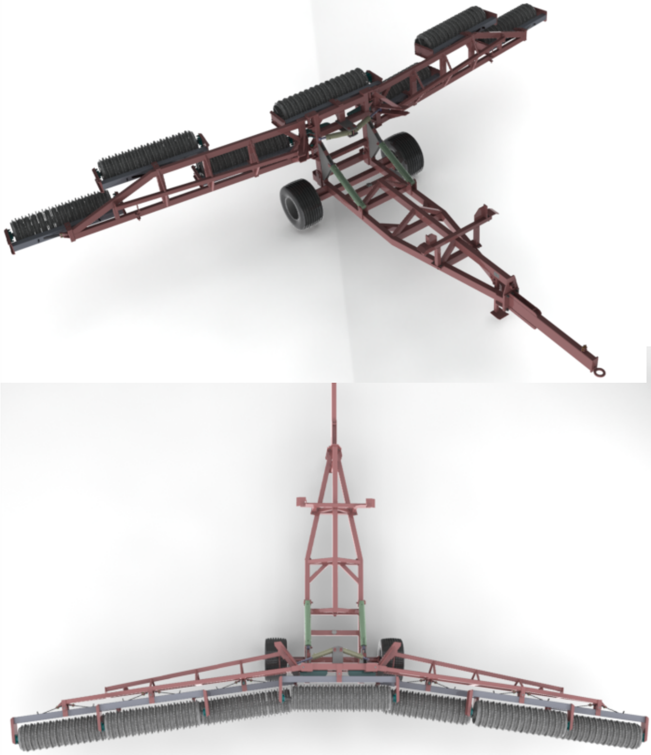
Рис. 11 Разведение крыльев малыми цилиндрами
