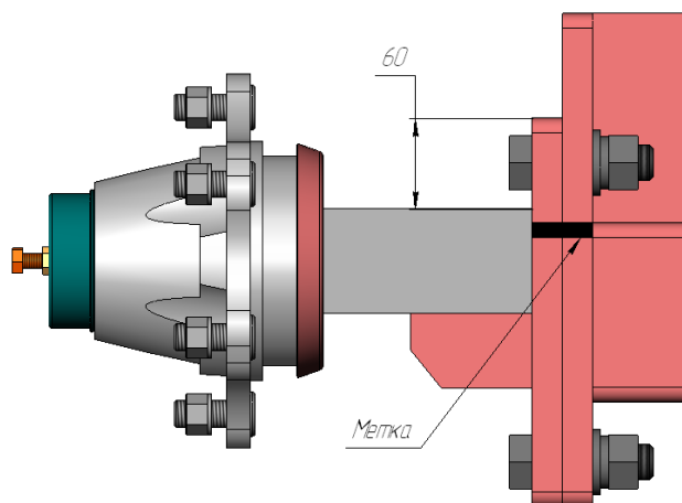
Рис. 5 Установка ступицы колеса
