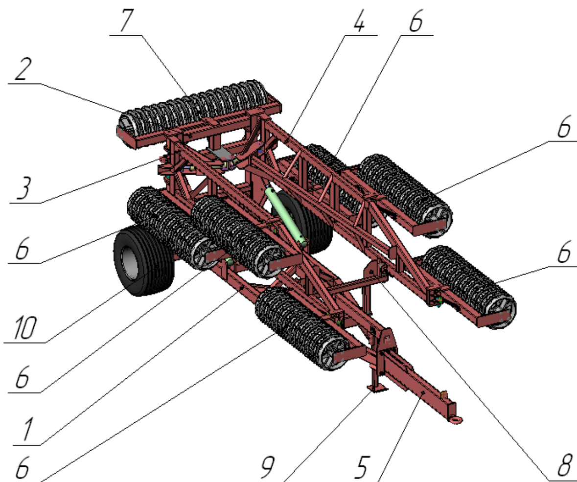
Рис.2 Общий вид катка кольчато-зубчатого Булава КЗ-12,4
